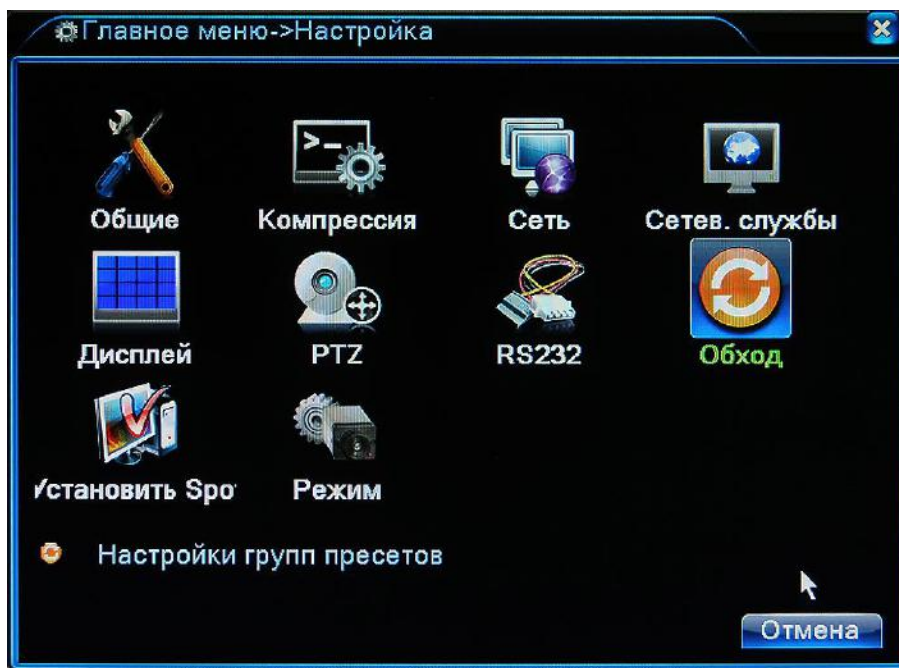
Рисунок 4.21 Настройка
