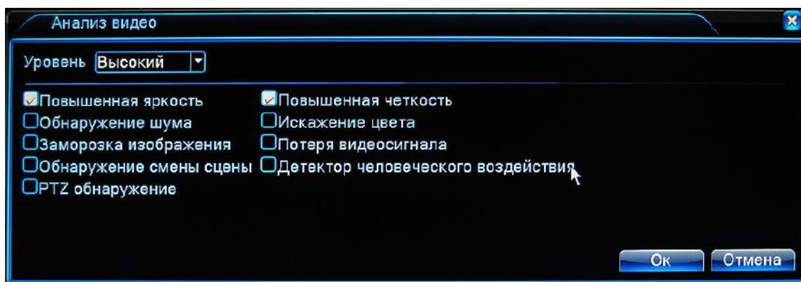
Рисунок 4.20 Анализ видео
