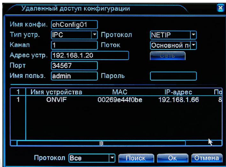
Рисунок 4.51 Конфигурация камер
