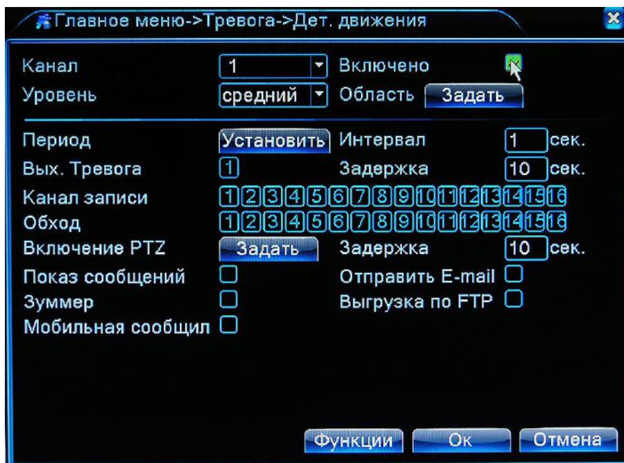
Рисунок 4.4 Детектор движения
