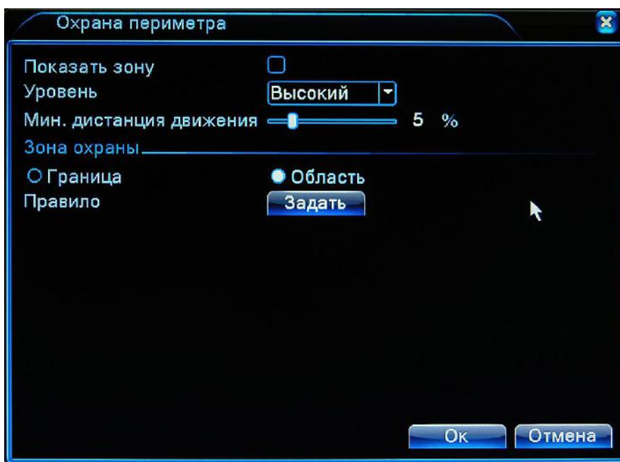
Рисунок 4.13 Охрана периметра
