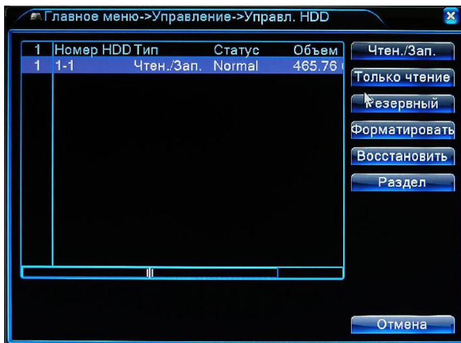
Рисунок 4.55 Управление HDD
