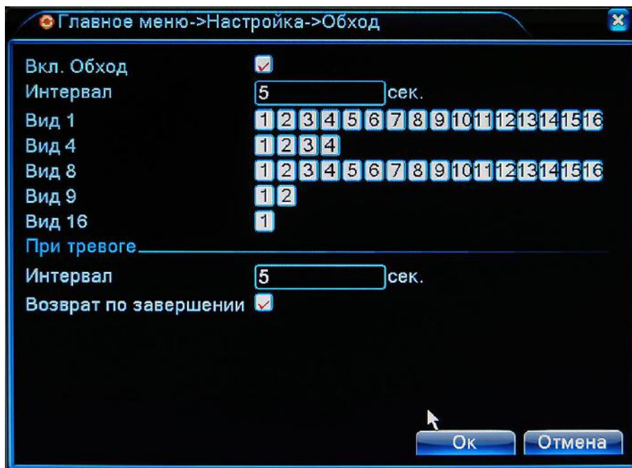
Рисунок 4.46 Обход
