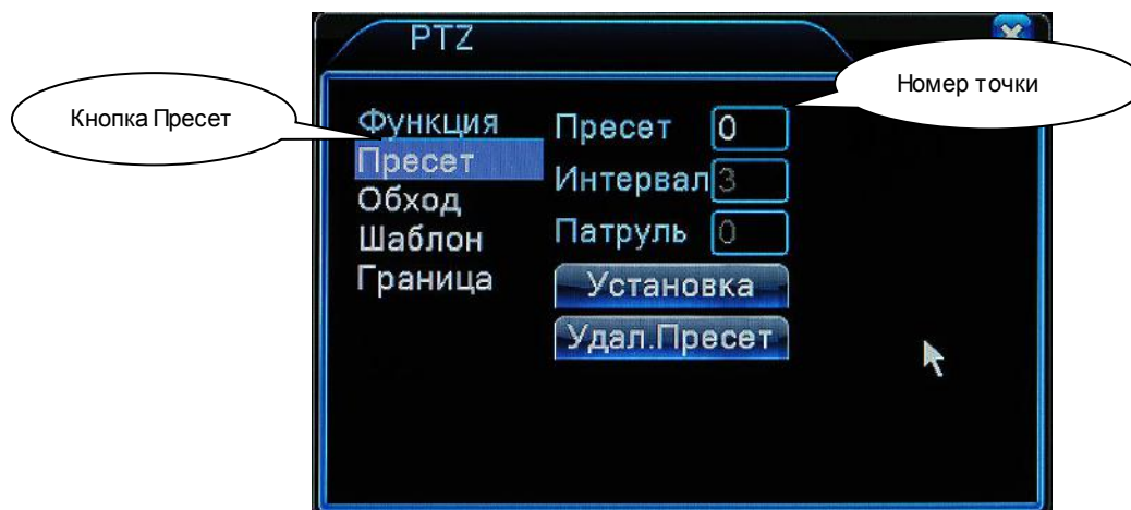
Рисунок 3.13 Настройка пресетов
