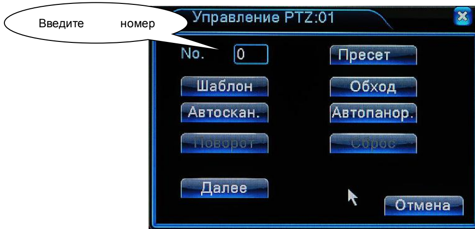
Рисунок 3.14 Управление PTZ
