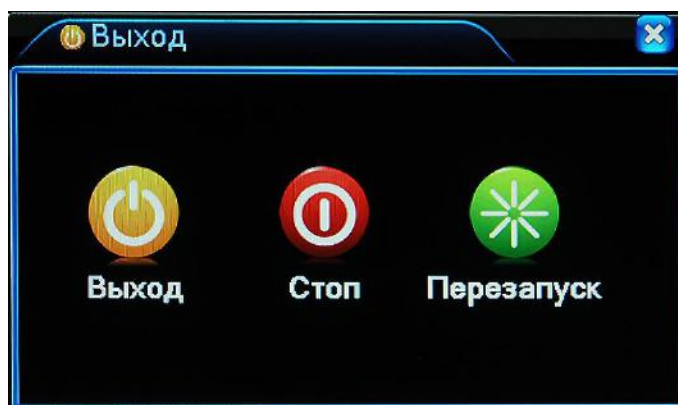
Рисунок 3.21 Выход/Стоп/Перезапуск
