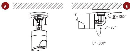
Рис. 5 Установка камеры Н1Т 13|Н1Т 23|Н1Т 53 на потолок
