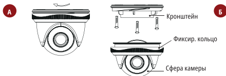
Рис. 3 Установка камеры Н1Т 12 | Н1Т 22 | Н1Т 52
