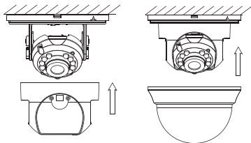
Рис. 2 Установка камеры Н1Т 10 | Н1Т 20 на потолок
