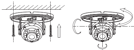
Рис. 1 Установка камеры Н1Т 10|Н1Т 20 на потолок
