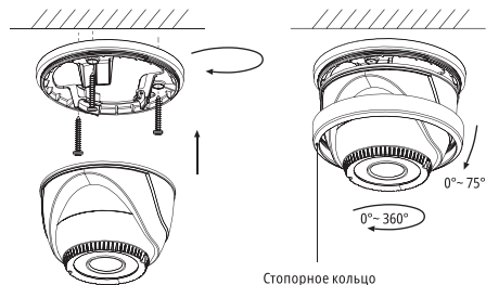
Рис. 6 Установка камеры Н1Т 27
